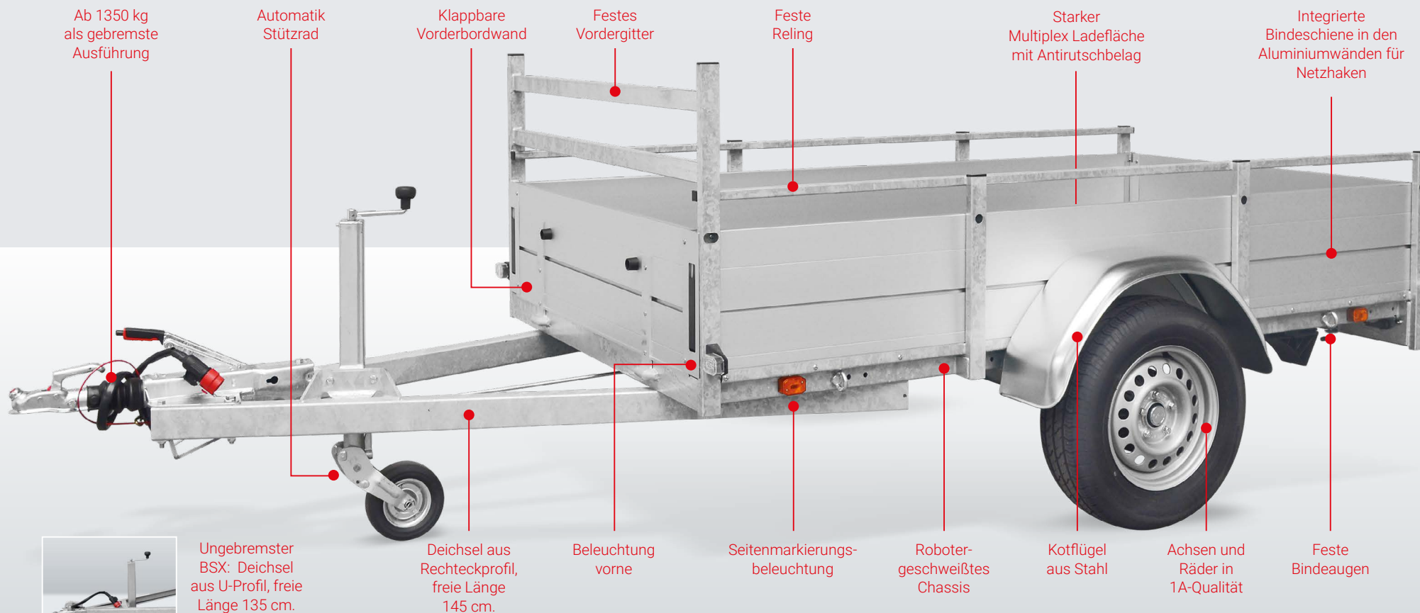
Robotergeschweißtes Chassis mit fester Reling und Vorgitter
