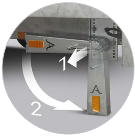
Zubehör: Abstellstützen
