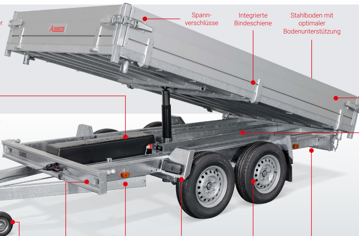
Automatik Stützrad
