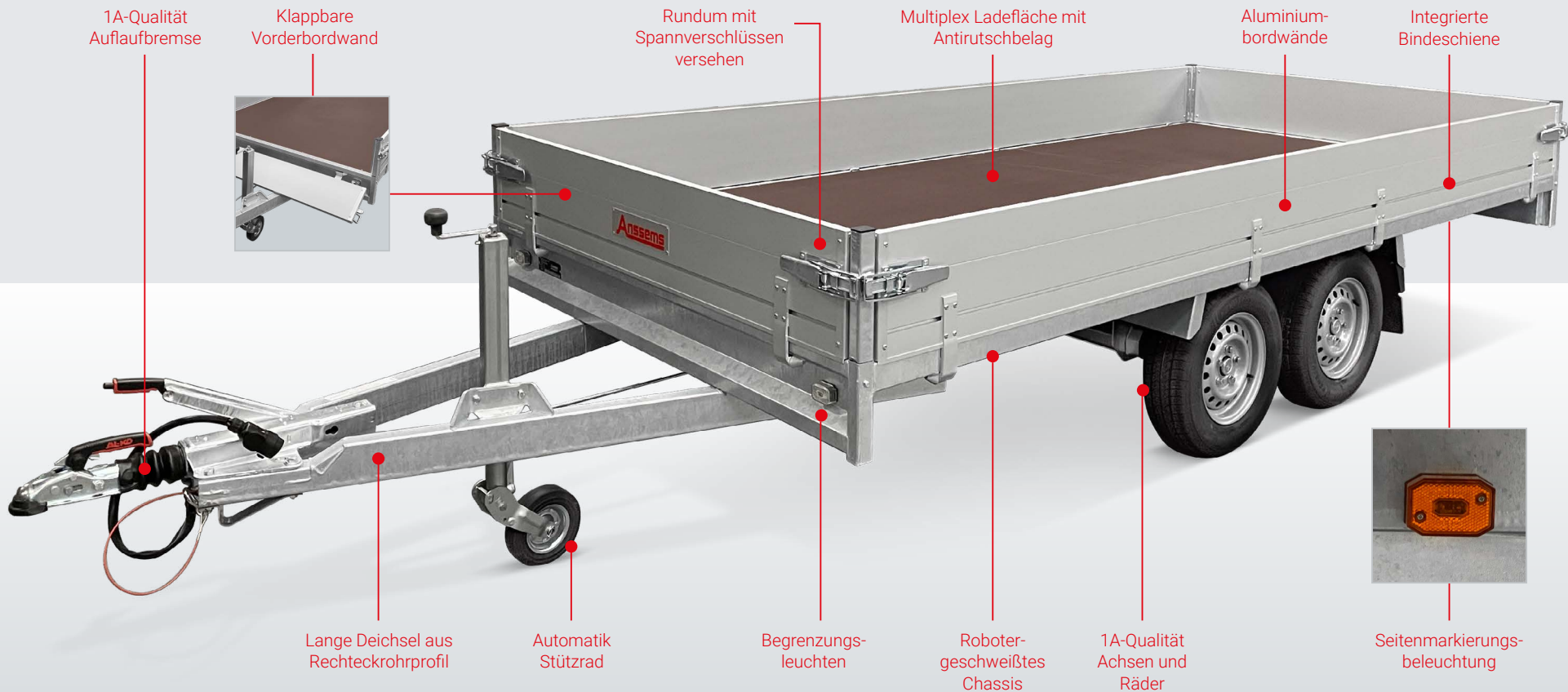
Bordwände klappen bis unter die Ladefläche. Beschädigungsfreies Be- und Entladen
